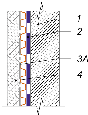
Защита тепло- и гидро-изоляционных материалов и пристенный дренаж
