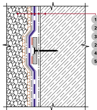
2. Крепление гидроизоляции на стенах тоннеля. Для крепления профилированной мембраны к гидроизоляции можно использовать полосы из применяемой гидроизоляционной мембраны.
