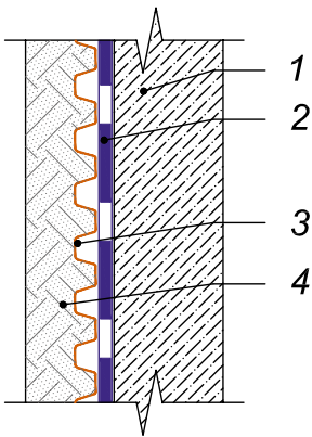
Защита гидроизоляционного материала на вертикальных конструкциях
