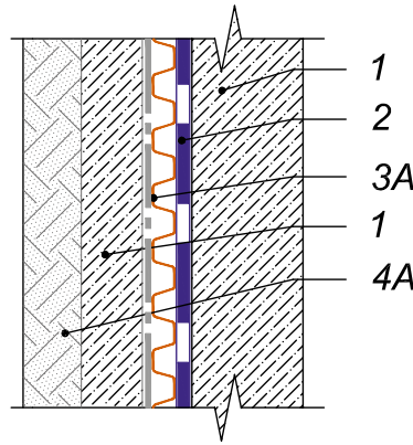
Защита стен фундаментов от подземных вод при строительстве способом «стена в грунте»
