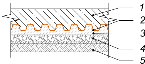
Конструкция пластикового дренажа и замена бетонной подготовки
