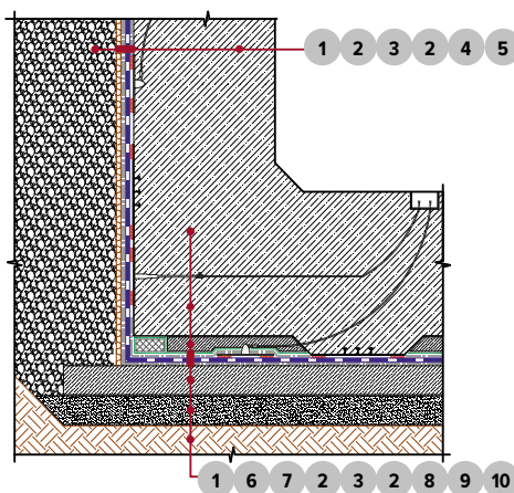
1. Гидроизоляция лотковой плиты в месте примыкания стены. Ориентация выступов при установке защитно-дренажных мембран PLANTER – к гидроизоляционному покрытию.
