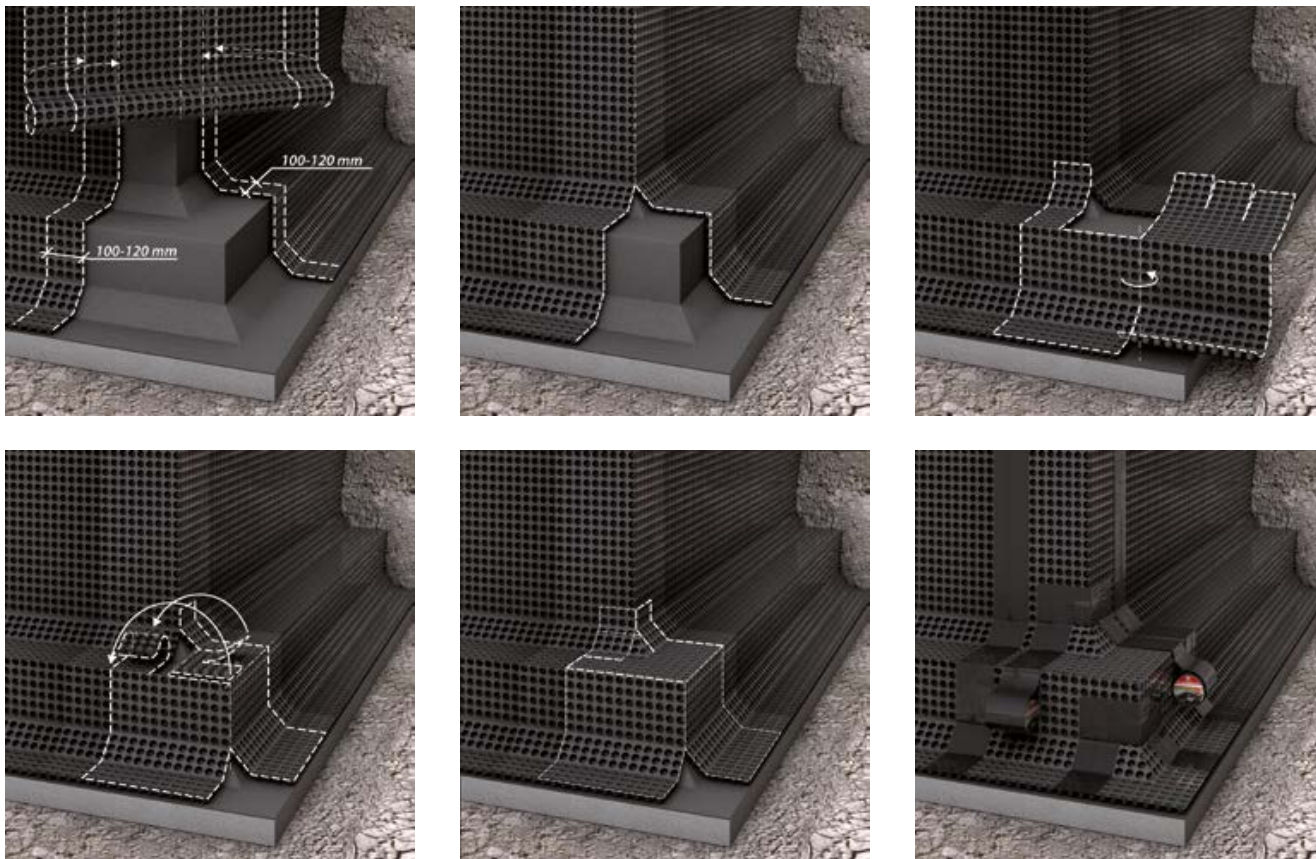
Рис. 2. Детали монтажа профилированных мембран на внешних и внутренних углах стены
