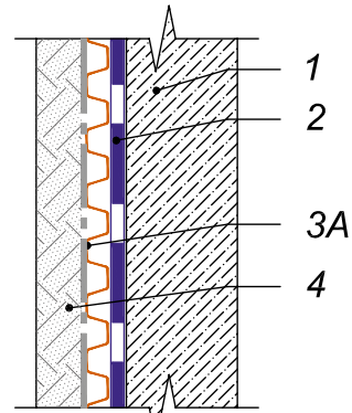
Защита гидроизоляционного материала и пристенный дренаж
