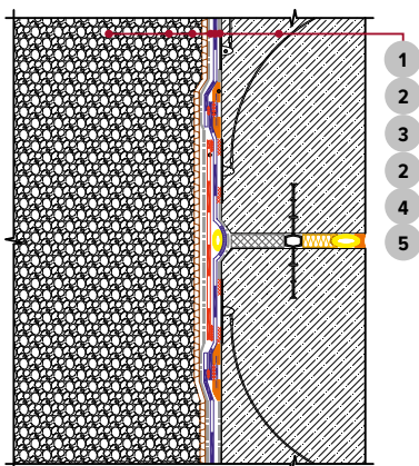
3. Деформационный шов. Формируйте дополнительный слой усиления гидроизоляционного покрытия в месте расположения деформационного шва.
