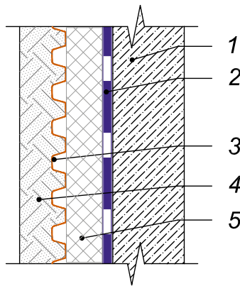
Защита тепло- и гидро-изоляционных слоев на вертикальных конструкциях
