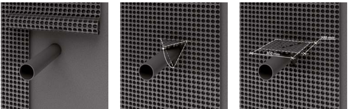
Рис. 3. Детали монтажа профилированных мембран в месте прохода коммуникаций
