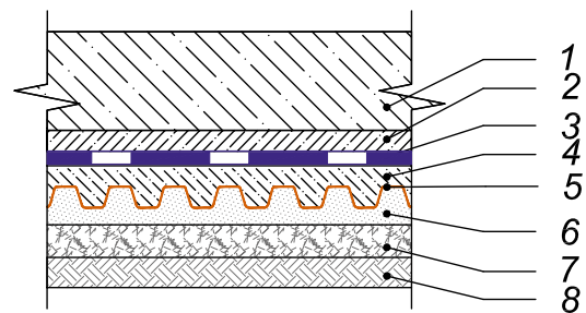
Конструкция пластикового дренажа в условиях высокого уровня грунтовых вод
