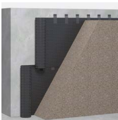
Рис. 5. Схема организации монтажа защитно-дренажных мембран PLANTER при высоте строительных конструкций более 4 м
