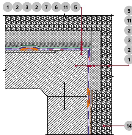
4. Гидроизоляция в верхней части стеновой конструкции. Для крепления мембраны PLANTER к экструзионному пенополистиролу используйте крепеж ТЕХНИКОЛЬ тип R.
